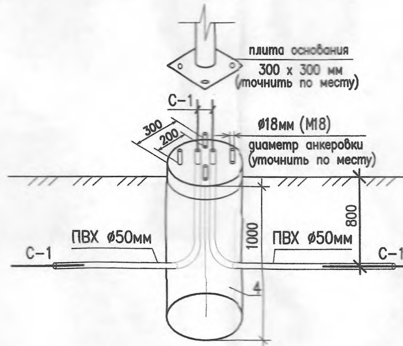
Установка опоры на бетонный фундамент Fm2a.
