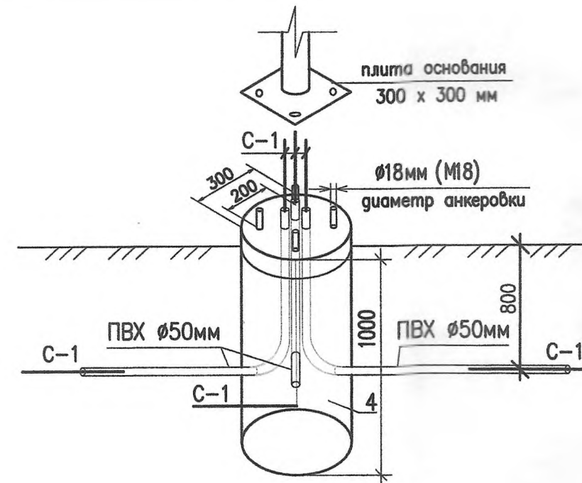
Установка опоры на бетонный фундамент Fm2.
