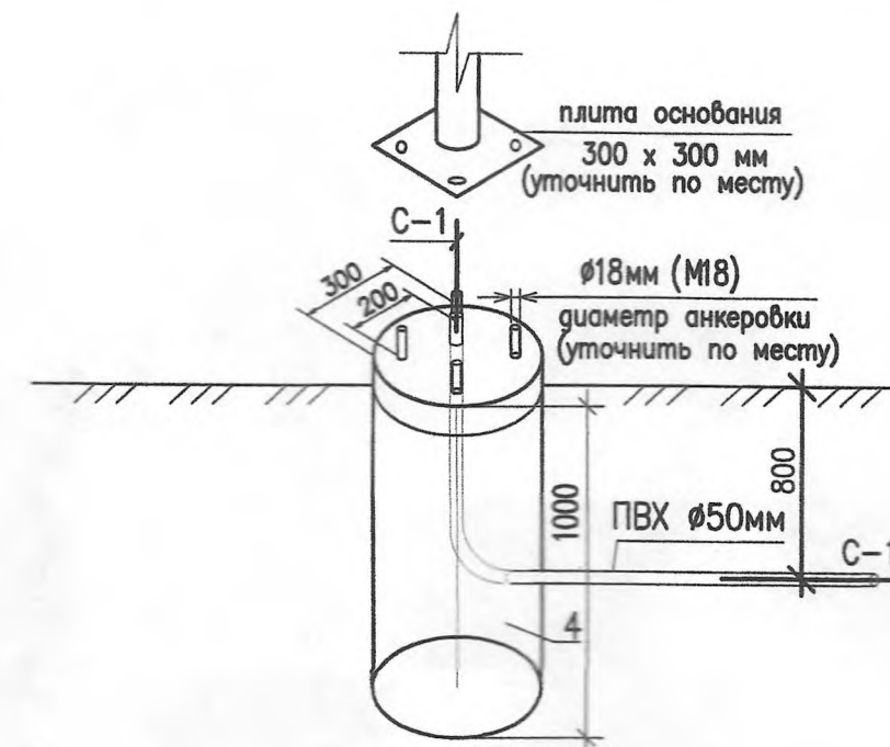
Установка опоры на бетонный фундамент Fm2b.
