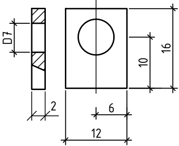
Detaliu poz.4
