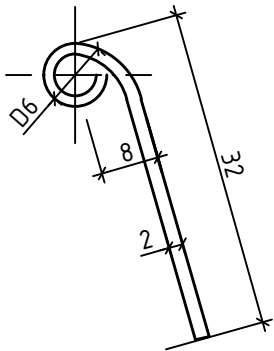
Detaliu poz.3
