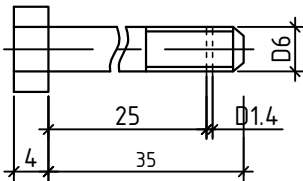
Detaliu poz.5
