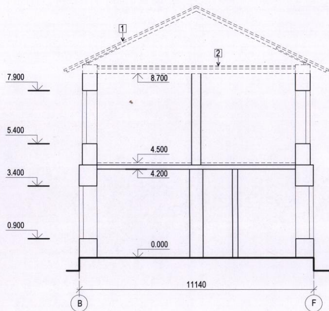
Sectiunea 3 - 3 demontare ( Releveu )
