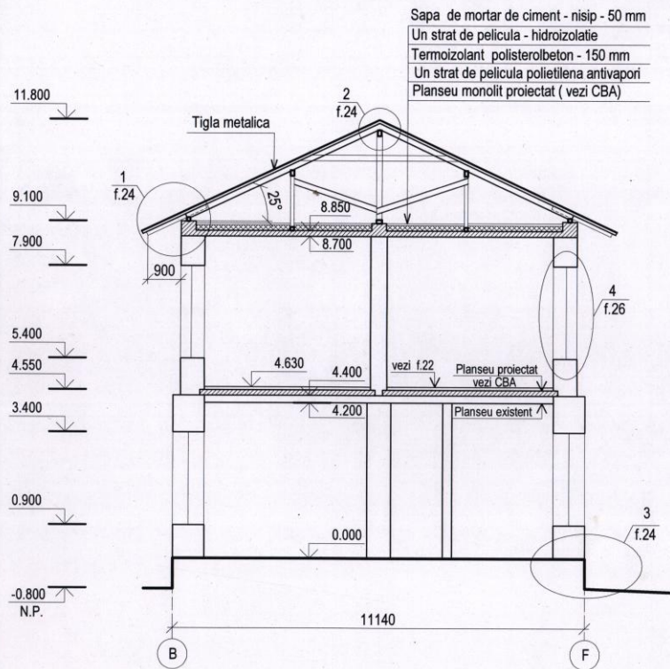
Sectiunea 3 - 3
