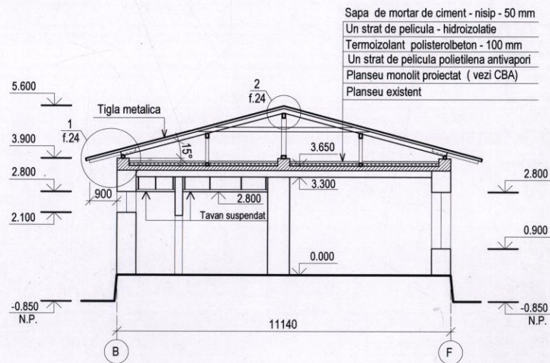
Sectiunea 4 - 4
