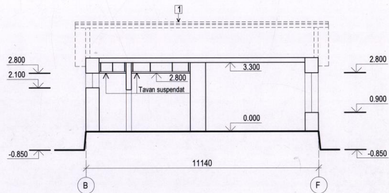
Sectiunea 4 - 4 demontare ( Releveu )
