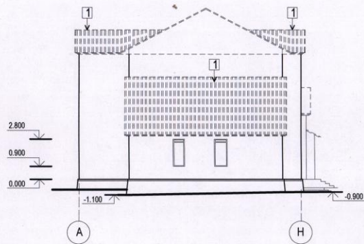
Fatada A - H demontare ( Releveu )
