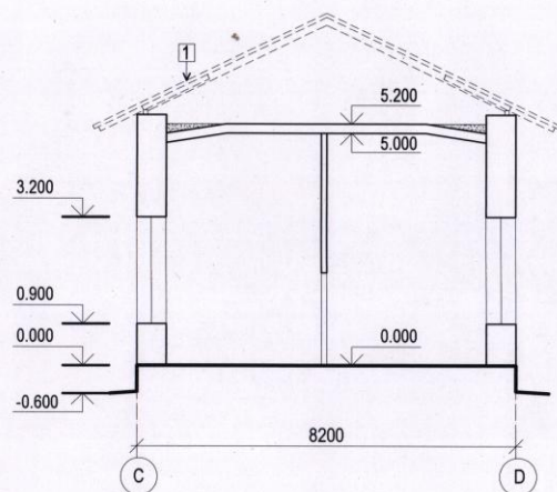
Sectiunea 2 - 2 demontare ( Relevu )
