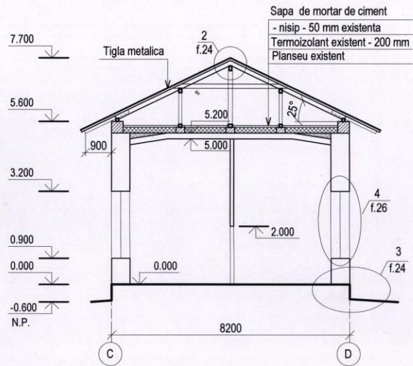
Sectiunea 2 - 2
