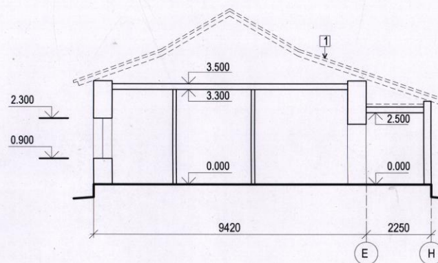
Sectiunea 1 - 1 demontare ( Relevu )
