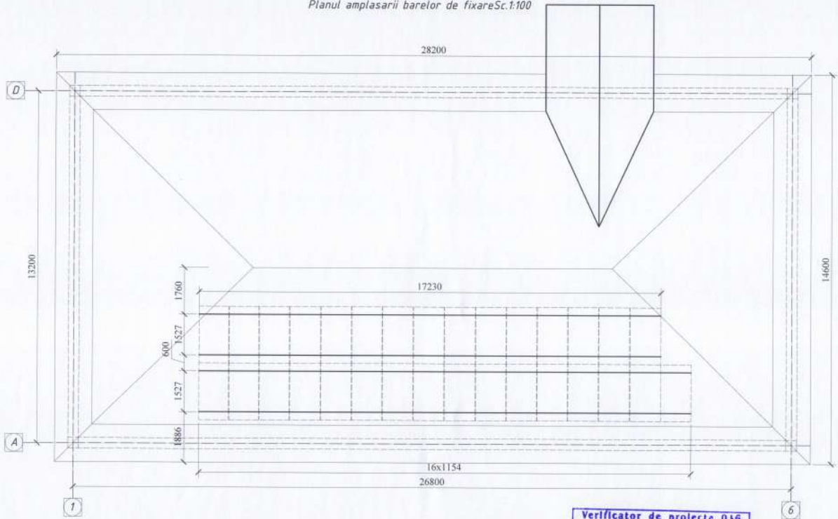
Planul amplasarii barelor de fixareSc.1:100
