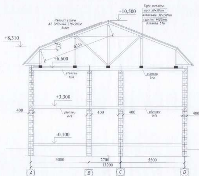
Sectiunea 1-1(relevu)Sc.1:100
