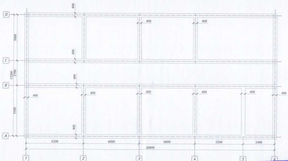
Planul amplasarii si peretilor portanti(relevu)Sc.1:100
