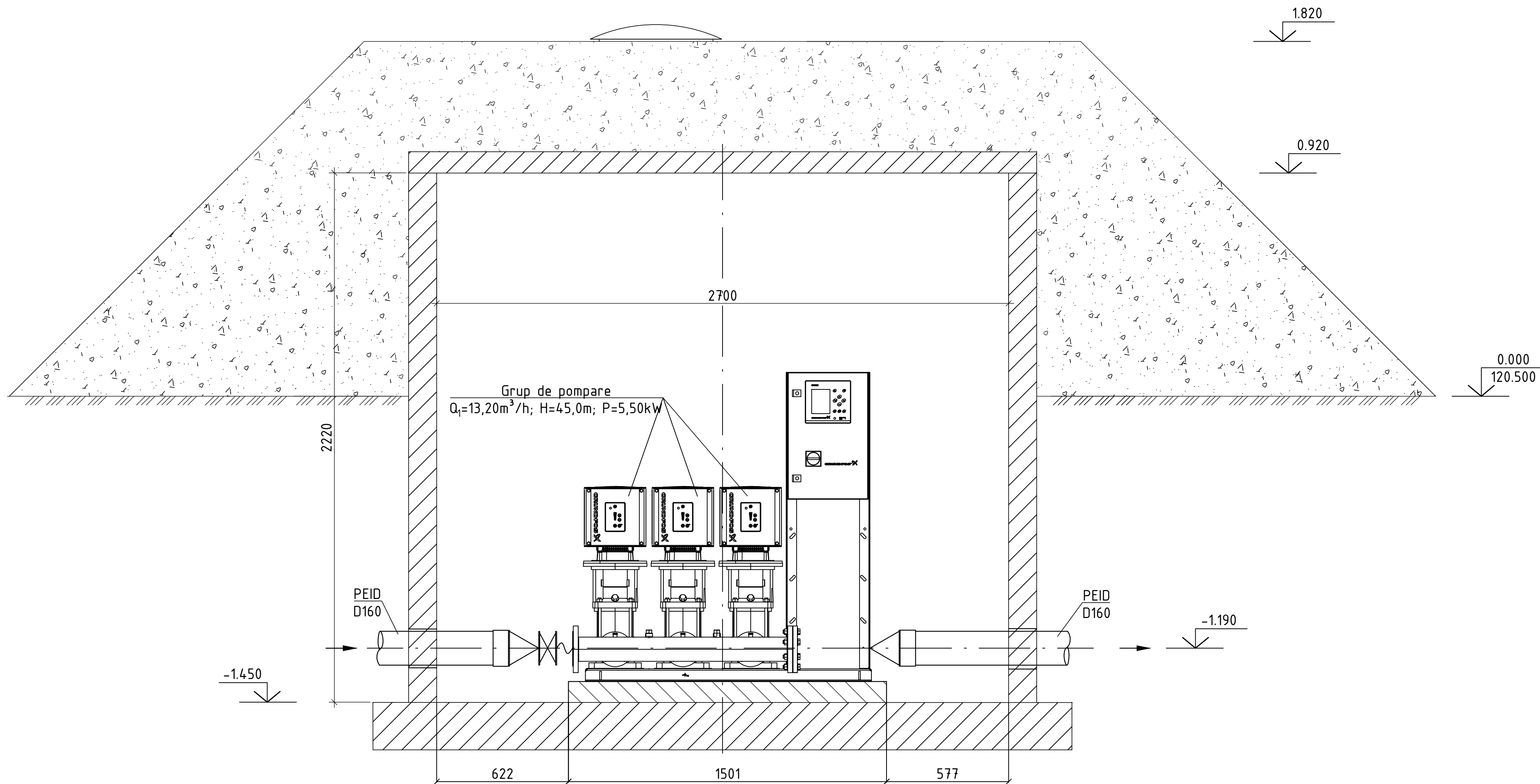
SECTIUNEA 2-2 Sc 1:20
