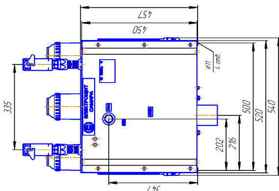
Рисунок А.1 – Габаритные, установочные и присоединительные размеры выключателя типа ВВУ-СЭЩ-ЭЗ-10. Тип подключения – два жгута с разъемами
