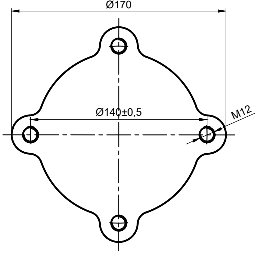
'X' Bakışı View 'X'
