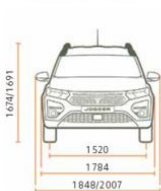
VEDERE FRONTALĂ
