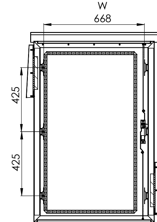
KESIT H-H ÖLÇEK 1 : 15
