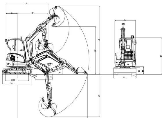
SCHEMA DIMENSIUNILOR ȘI RAZA DE ACȚIUNE — Model R32
