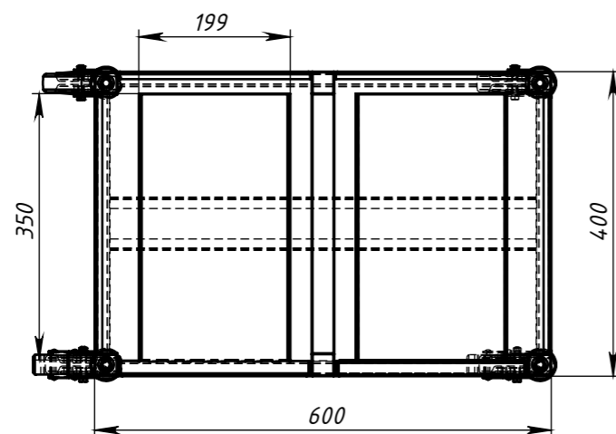
A-A (1 : 9)
