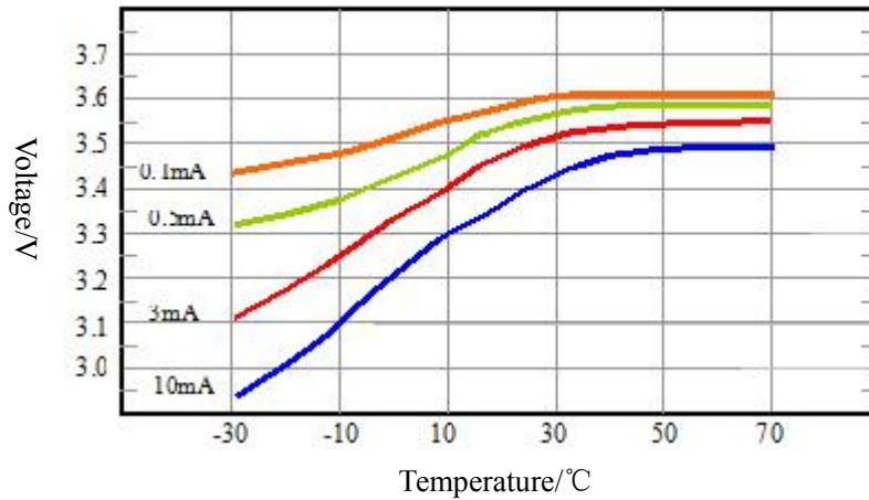
不同温度下电压平台特性图
