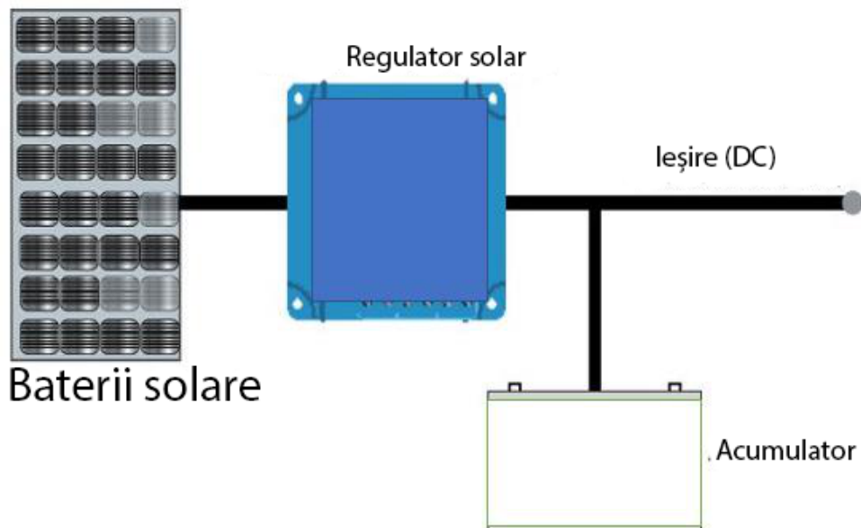
Figura1. Schema centralei autonome de curent continuu.
