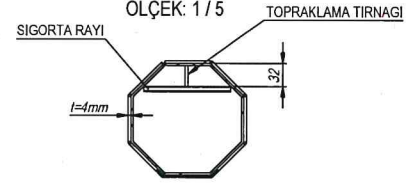
KESİT S-S ÖLÇEK 1:5
