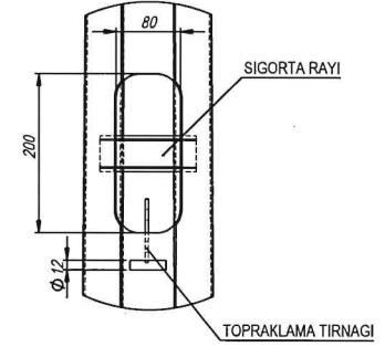
DETAY P ÖLÇEK: 1/5
