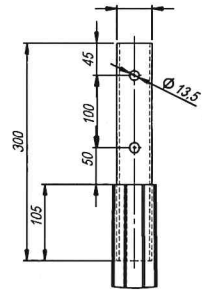
DETAY Q ÖLÇEK: 1/5
