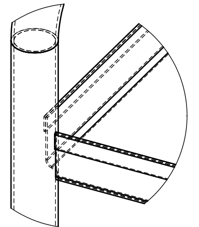
B (1 : 2)
