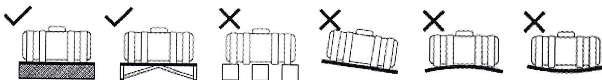
Рис.2 – Схематичне зображення монтажу ємності.
