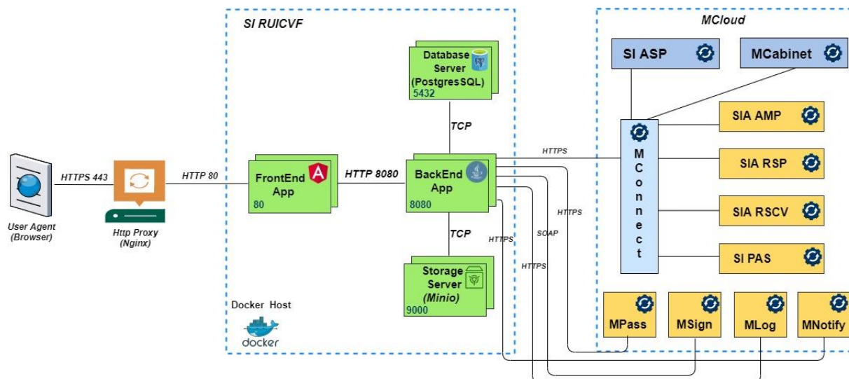
Figura 1. Arhitectura SI RUICVF.
