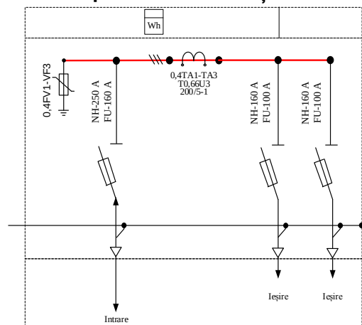
245 nr. 1. Schema monofilară a PPDÎTV cu aparate de comutație
