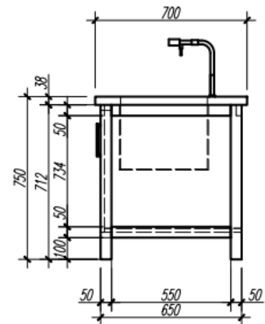
Masa de laborator cu chiuveta incorporabila L=1200x700x750
