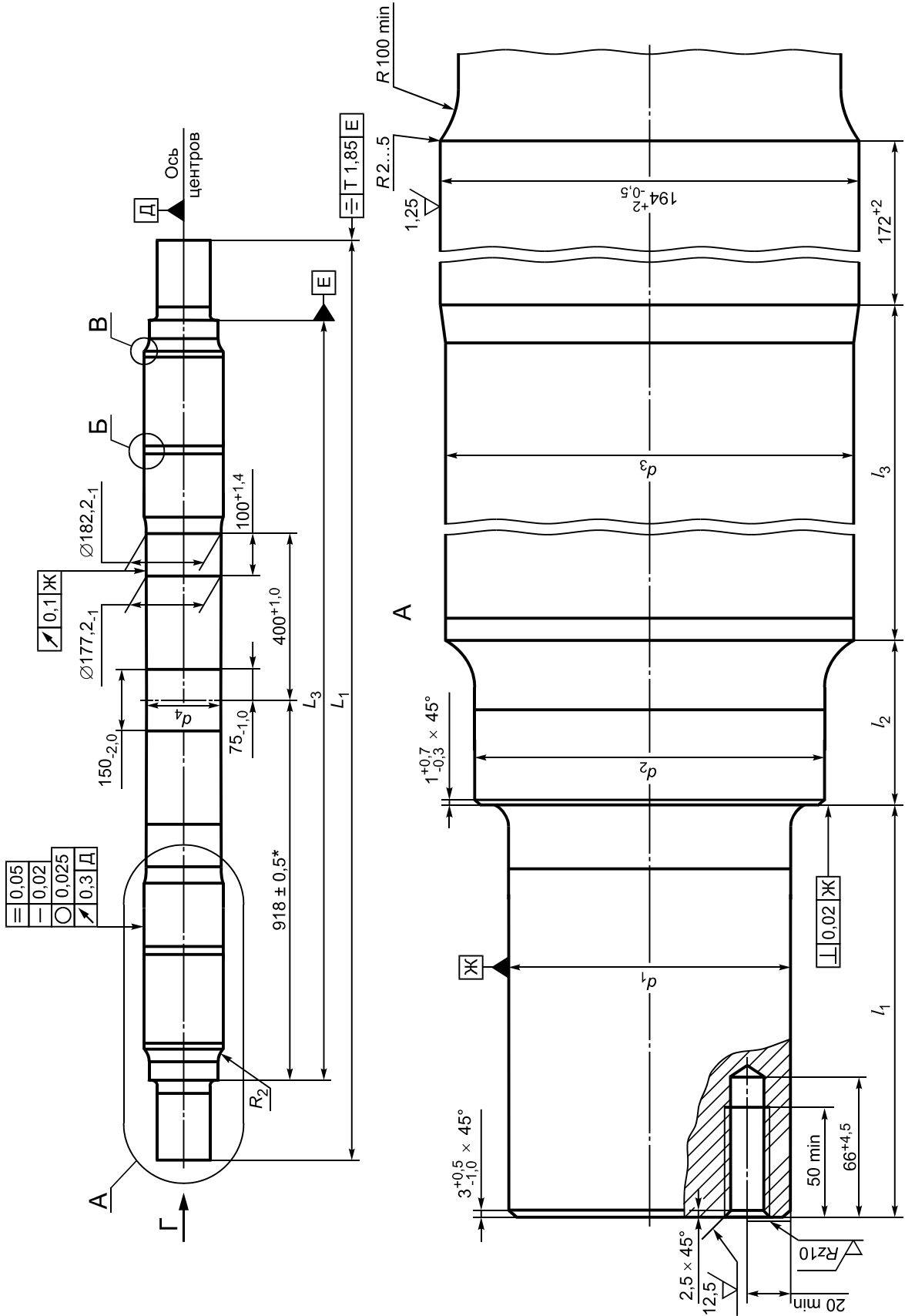
Рисунок А.5, лист 1 — Ось типа РВЗШ для пассажирских вагонов локомотивной тяги, СПС
