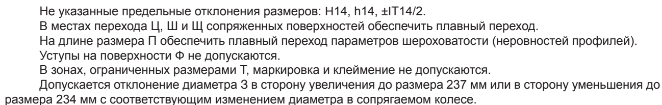
Рисунок А.8, лист 2 — Ось для электровозов ЭП2К
