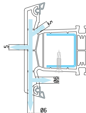
горизонтальный импост
