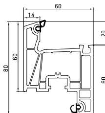
Створка 4-камерная 025
