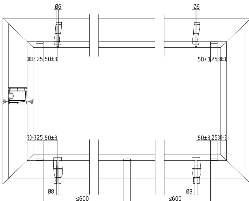
Ширина створки более 600мм
