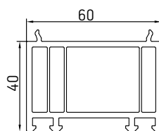
013 Расширитель рамы 40/60
