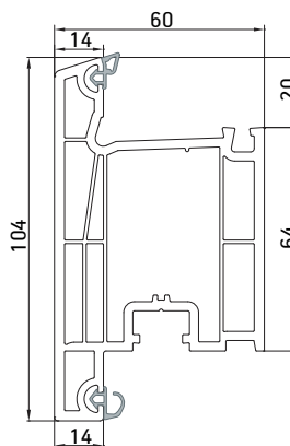
Дверная створка внутреннего открывания
