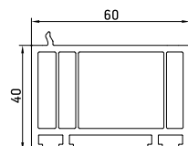
Соединитель-усилитель 035
