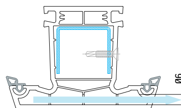
вертикальный импост
