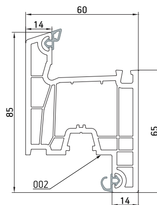
Створка 4-камерная
