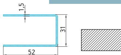
Дверная створка с металлом U31/52/1,5
