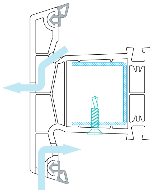
Рис. 4. Типовые схемы вентиляции импоста
