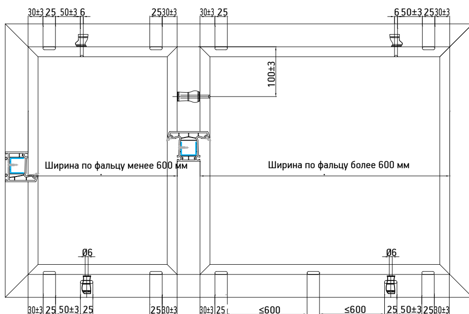
Отверстия в раме с импостом
