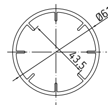
034 Подоконный профиль
