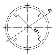
Круговой коннектор 010
