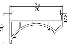
Адаптер кругового коннектора 70 053
