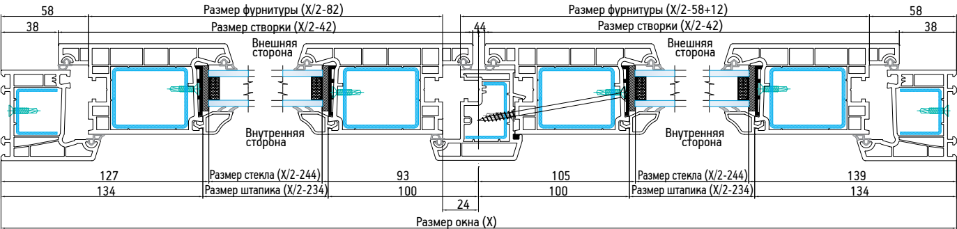
A-A
