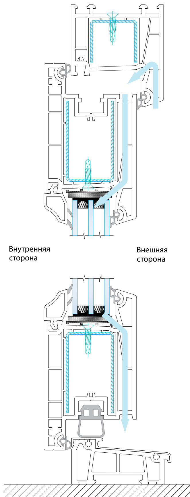
Рис.36 Типовые схемы вентиляции дверной створки
