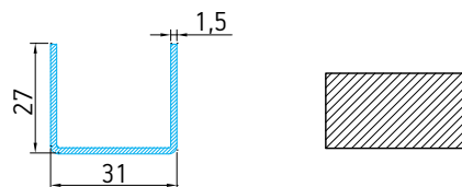
Створка 4-камерная с металлом U31/27/1,5
