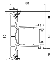
Импост 4-камерный 027
