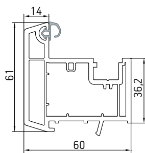
012 Штульп 60 мм
