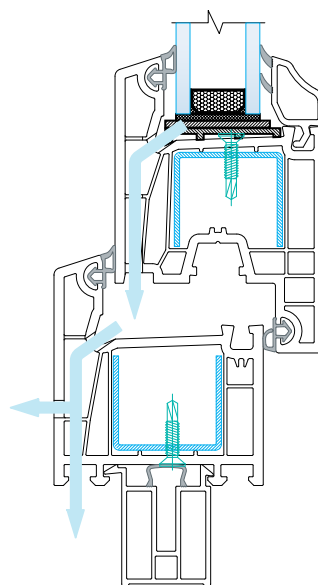
Рис. 2. Типовые схемы вентиляции
