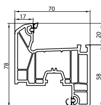
Створка 5-камерная 062
