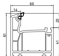
Рама 4-камерная 037
