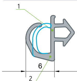
Уплотнитель створки
