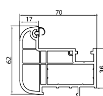
Штульп 70мм 054
