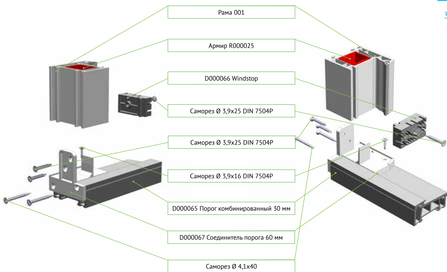
Рис. 116. Схема монтажа рамы с порогом
