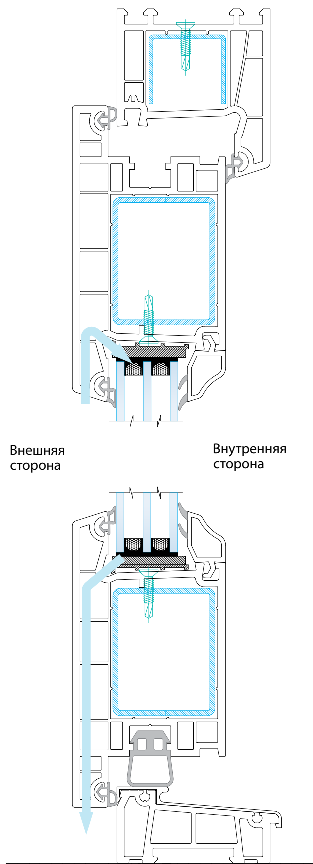
Рис.3в Типовые схемы вентиляции дверной створки
