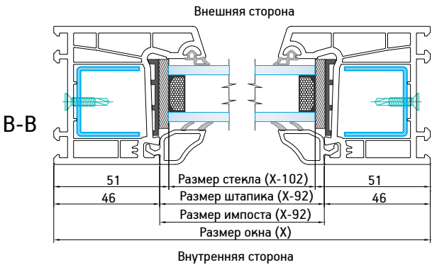
Внутренняя сторона
