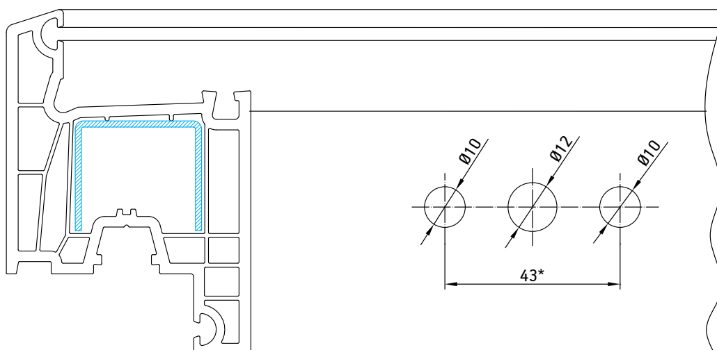
Рис. 1. Фрезеровка и сверление отверстий для установки фурнитуры
