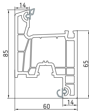
002 Створка 4-камерная
