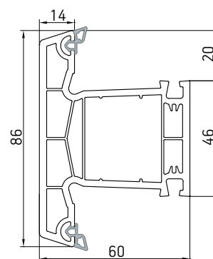
003 Импост 4-камерный
