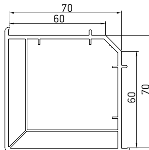
023 Уловой соединитель 90°
