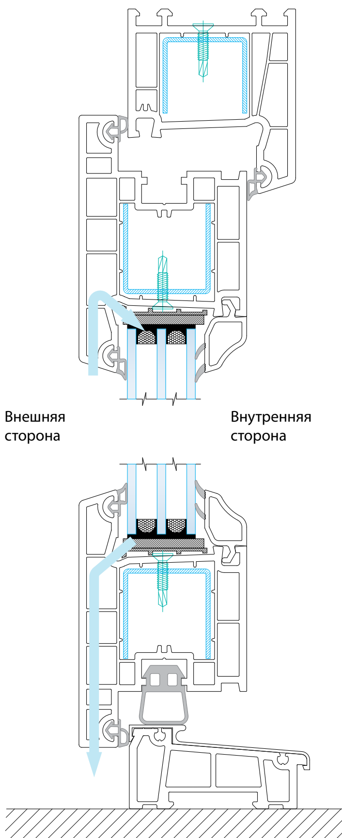
Рис.3г Типовые схемы вентиляции дверной створки
