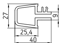
035 Соединитель-усилитель
