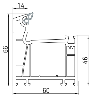
001 Рама 4-камерная
