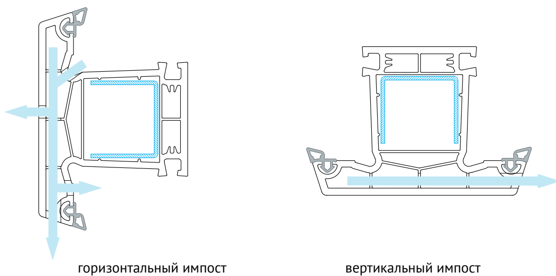
Рис. 7. Типовые схемы вентиляции предкамеры для цветных профилей
