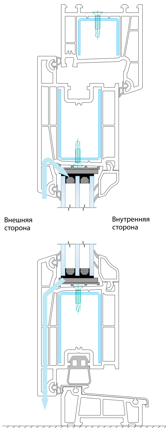
Рис.3а Типовые схемы вентиляции дверной створки
