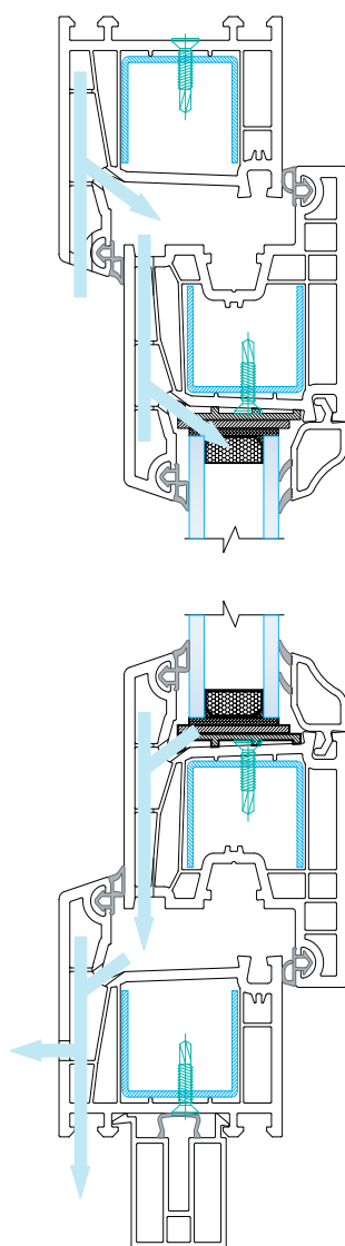
Рис. 6. Типовые схемы вентиляции предкамеры для цветных профилей
