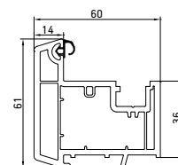
Штульп 60мм 012
