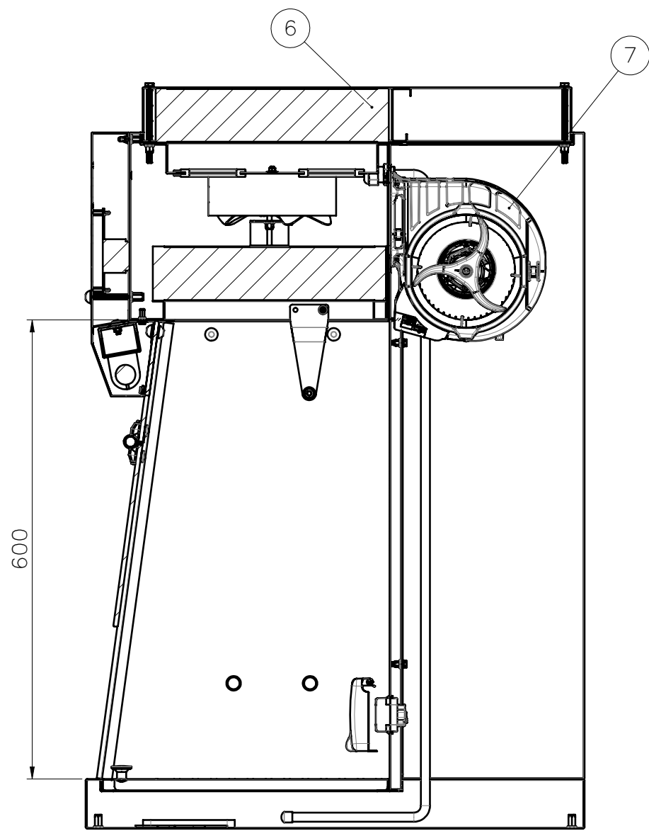
SEZIONE A-A
