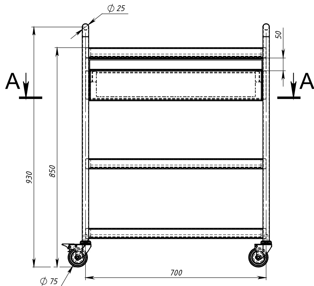
A-A (1 : 9)
