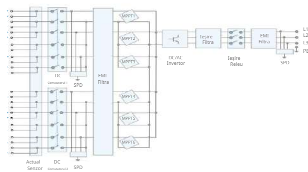
Schema circuitului
