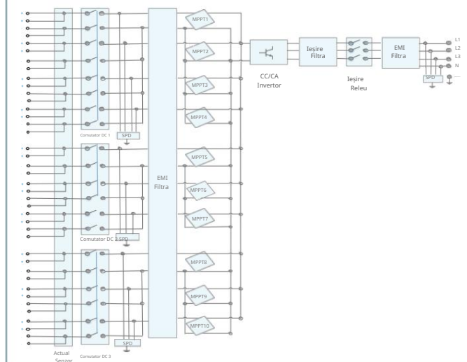
Schema circuitului
