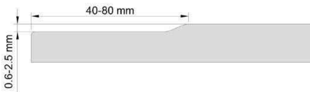
Muchie PRO – secțiune
