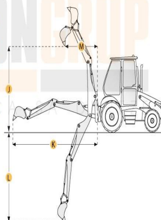
Figura 10. Caracteristicile tehnice CAT432E
