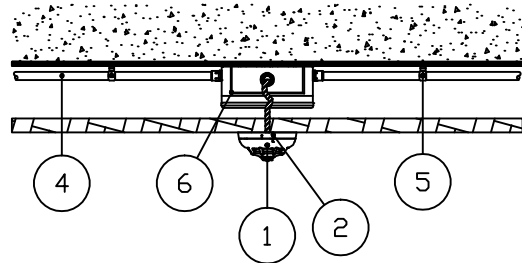
ПОТОЛОЧНАЯ УСТАНОВКА
