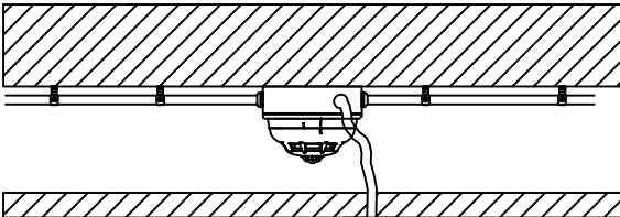
ПОТОЛОЧНАЯ УСТАНОВКА
