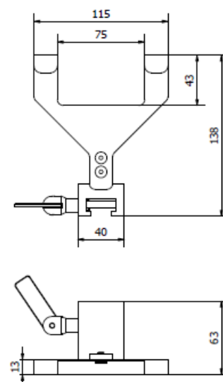
Heel holder (4-09-104)
