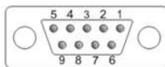
RS-232 DB9
