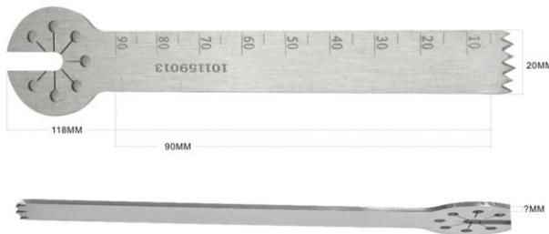
► SAW BLADE
