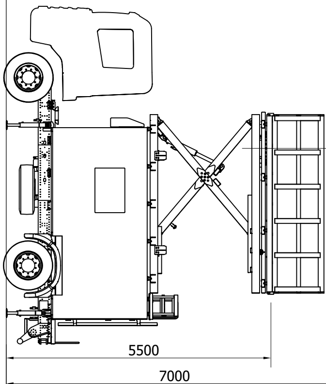
Pozitii nacela tip foarfeca
