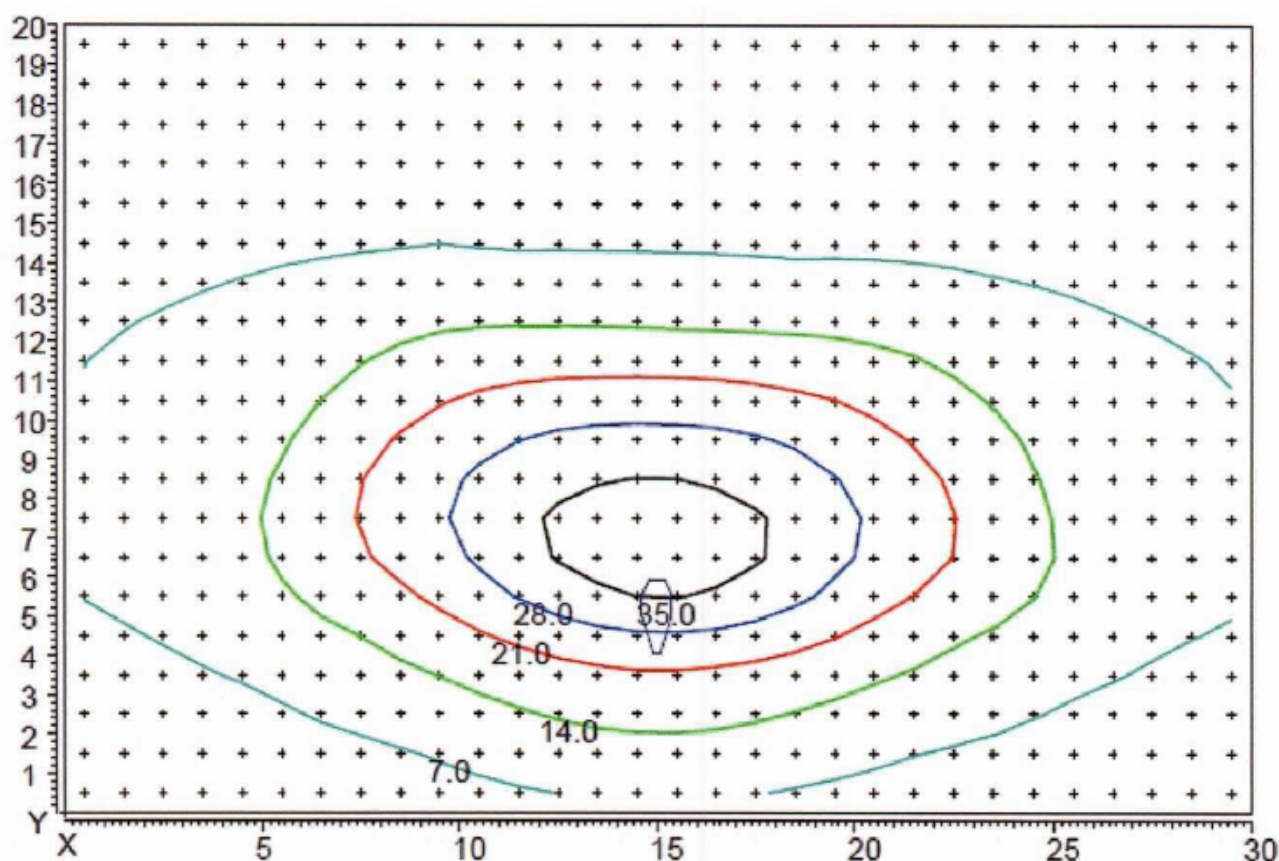
Distribuția luminii pentru înălțimea de fixare a corpului de 10 m.
