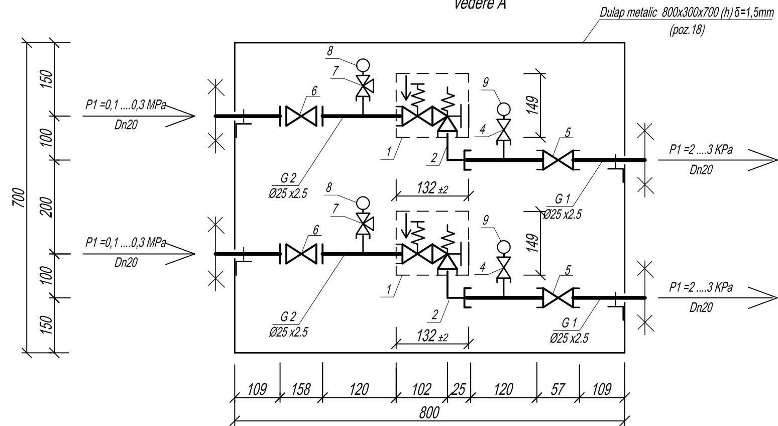
SCHEMA TEHNOLOGICĂ S 1:10 vedere A
