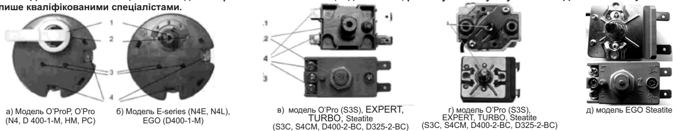
1 - регулятор температури, 2 - Кнопка теплового захисту, 3 - Гнізда підключення сигнальної лампи, 4 - Клеми підключення до електроенергії
