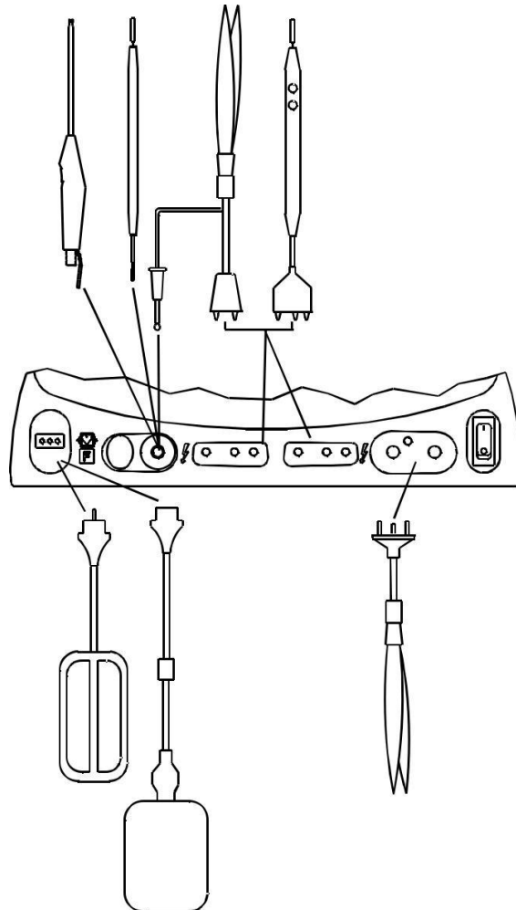
Figura 2.5 Conexiunile accesoriilor
