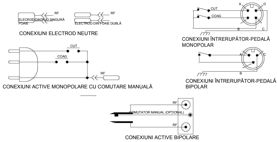
Figura 2.4 Schema de accesorii
