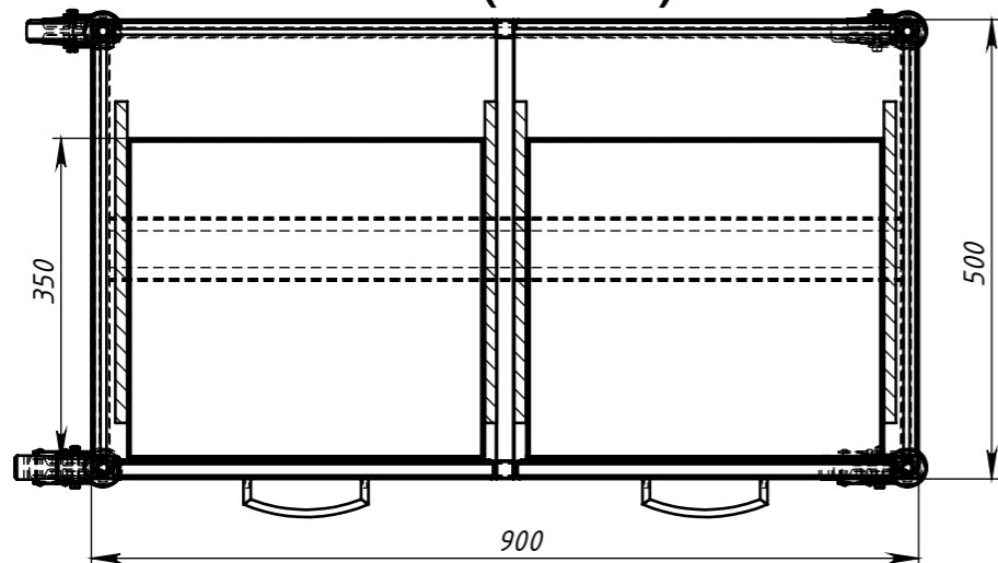
A-A (1 : 9)
