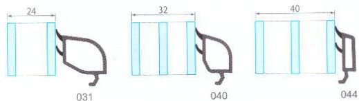
Штапики
