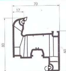
093 Створка 6-камерная Class A
