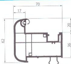
054 Штульп
