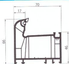
059 Рама 6-камерная
