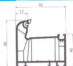
092 Рама 6-камерная Class A
