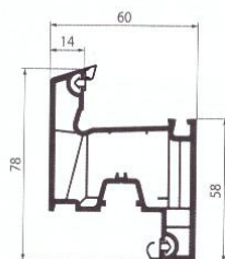
087 Створка 5-камерная
