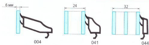
Штапики
