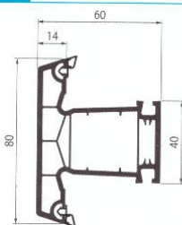
027 Импост 4-камерный
