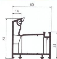
086 Рама 5-камерная
