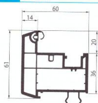
012 Стульп
