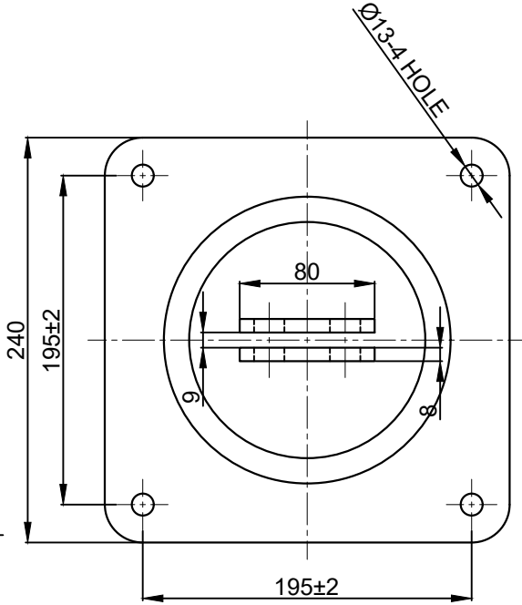
'X' Bakışı View 'X'
