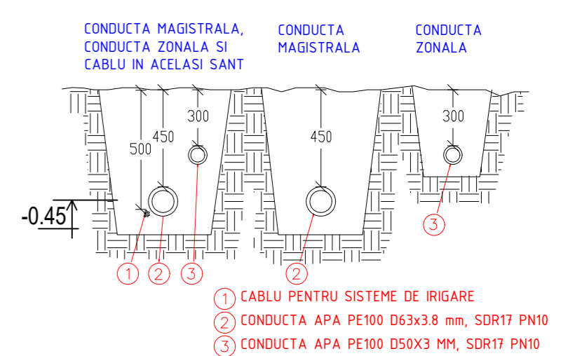
DETAILIU POZARE CONDUCTE SI CABLURI IN SANT
