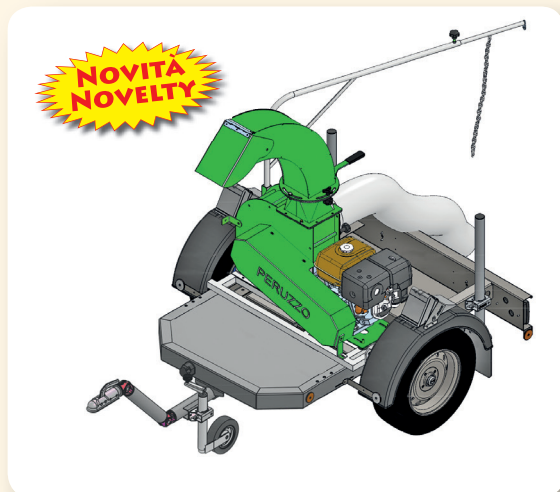
TURBO 400 su carrello stradale omologato TURBO 400 on approved road chassis TURBO 400 sur châssis routier approuvé TURBO 400 auf zugelassenem Straßenfahrgestell
