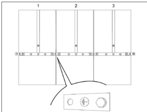
Рис. 4.38 Заземление оборудования
