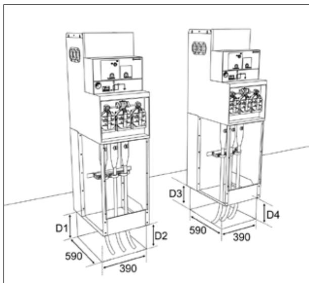
Рис. 4.5 Размеры [мм] кабельного колодца для cgmcosmos-p и cgmcosmos-a
