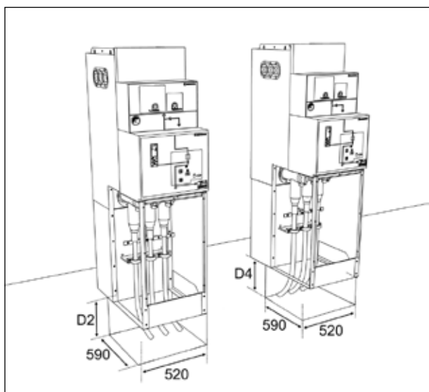
Рис. 4.6 Размеры [мм] кабельного колодца для cgmcosmos-с с приводным механизмом AV/RAV
