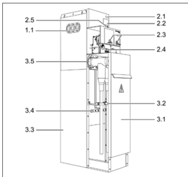
Рис. 1.1 Основные компоненты ячеек sgmcosmos
