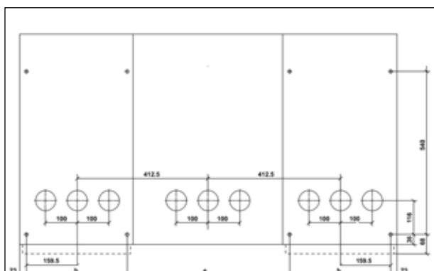
Рис. 4.26 Схема анкерного крепления cgmcosmos-2lp , -rlp высотой 1740 мм
