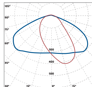
«Diora Unit PRO Ш2» широкая боковая КСС 130°x60°
