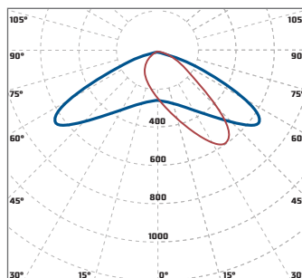
«Diora Unit Ш1» широкая КСС 140°x30°
