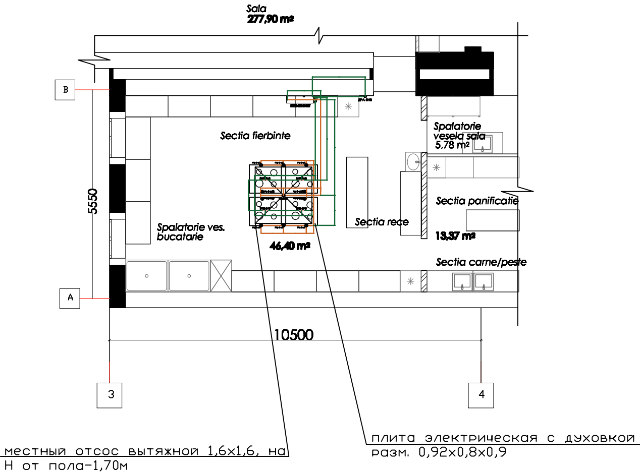
План размещения оборудования кухонного тушения.
