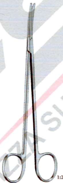
Toennis - Adson
