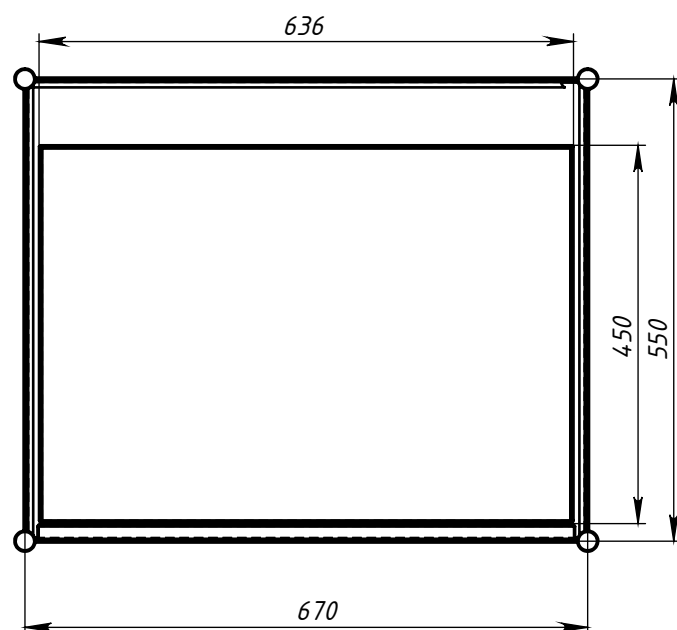
A-A (1 : 9)
