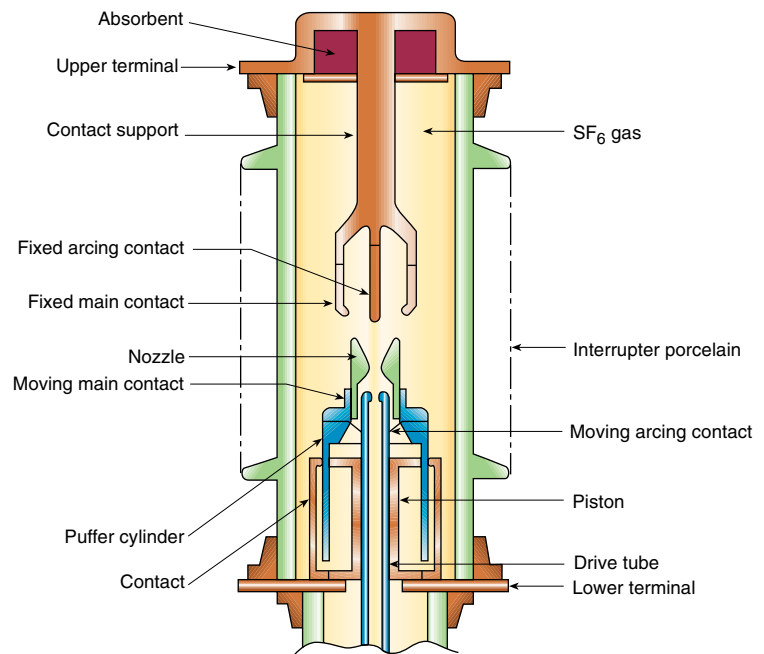
FIG. 2 : Open position
