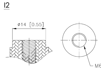
[M6 bolt]
