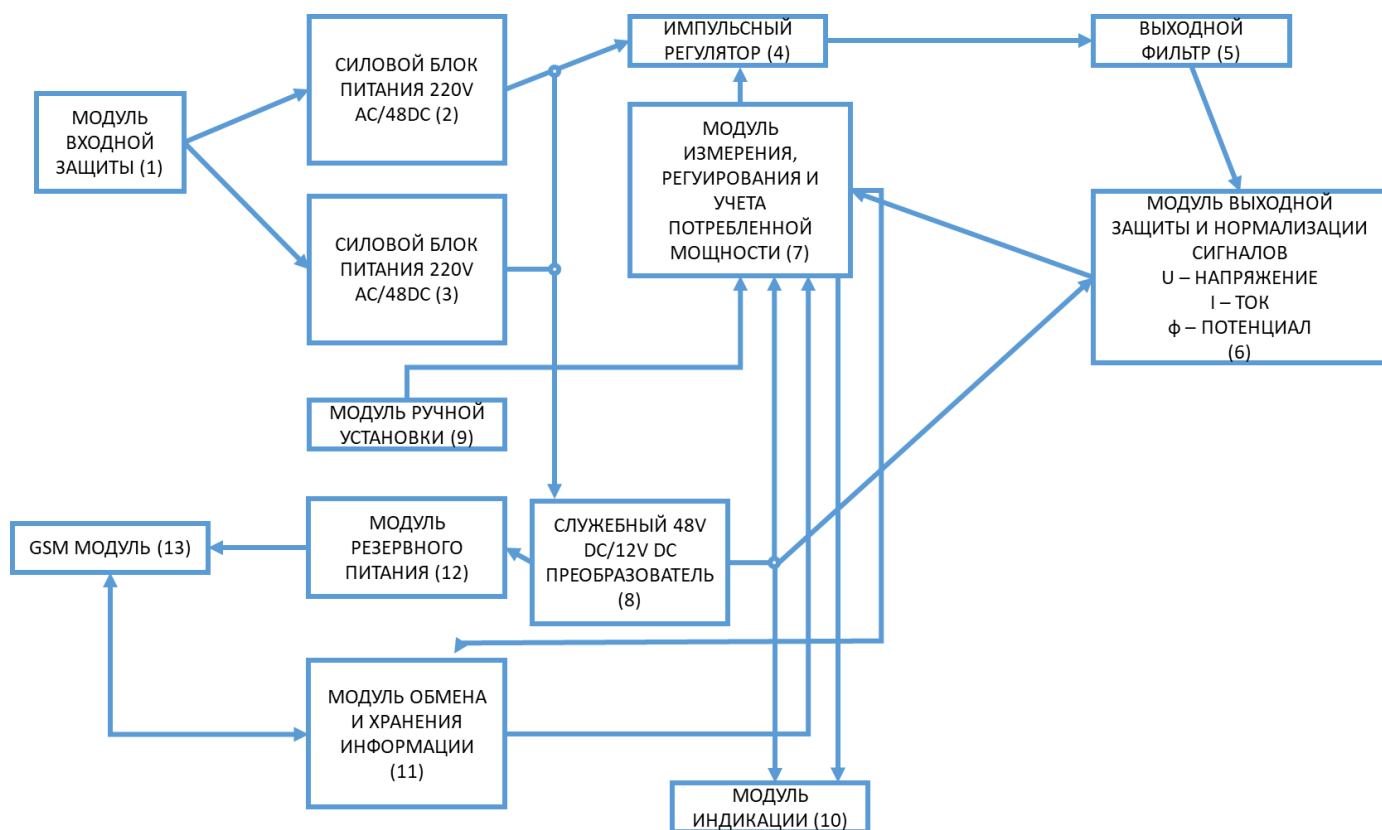
Рис.1 Блок схема станции катодной защиты.
