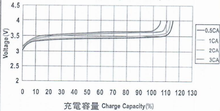
常溫下LYP類電池的充電特性曲綫
