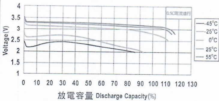
不同環境溫度下LYP類電池的放電特性曲綫
