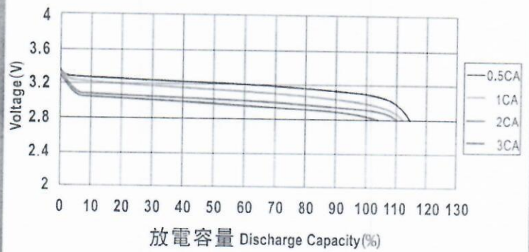
常溫下LYP類電池的放電特性曲綫
